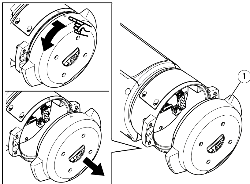
1 Монтажное основание
