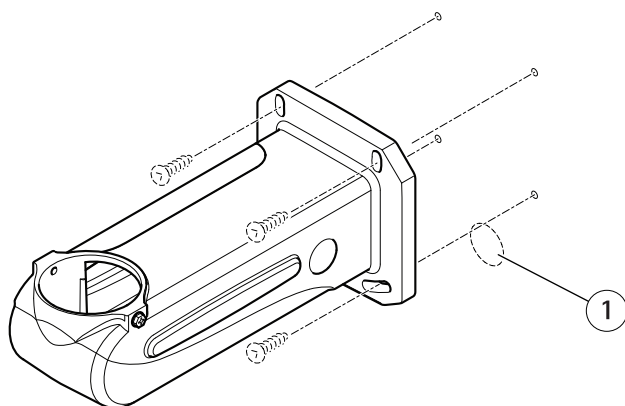
1 ケーブル孔
