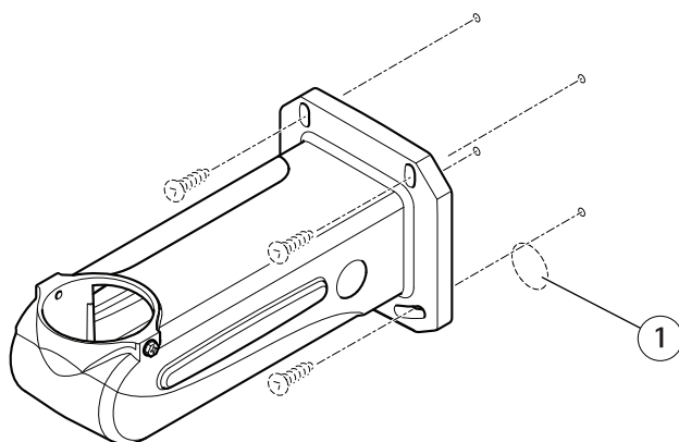
1 Kabeldurchführung
